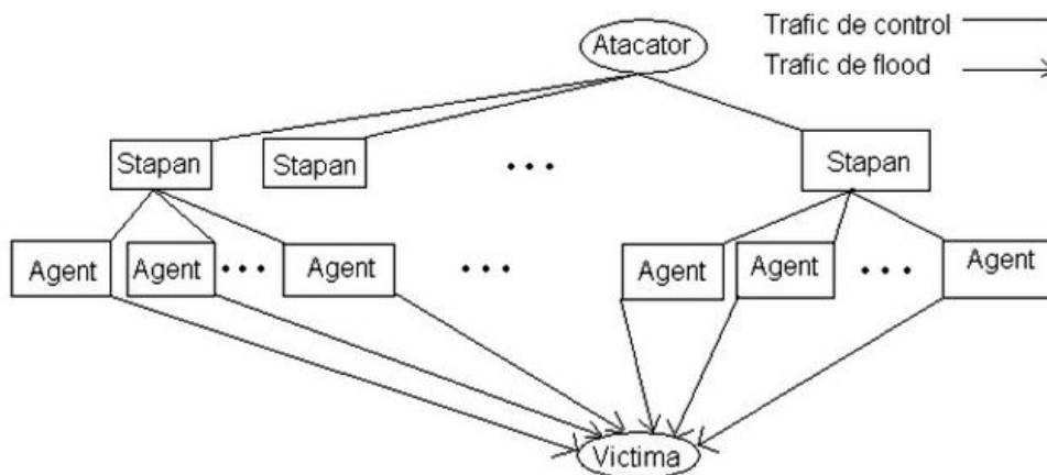
Fig. 2 Arhitectura unui atac DDoS
